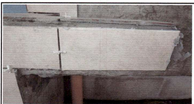
Foto 5: Instalación de azulejos en piletas de concreto
